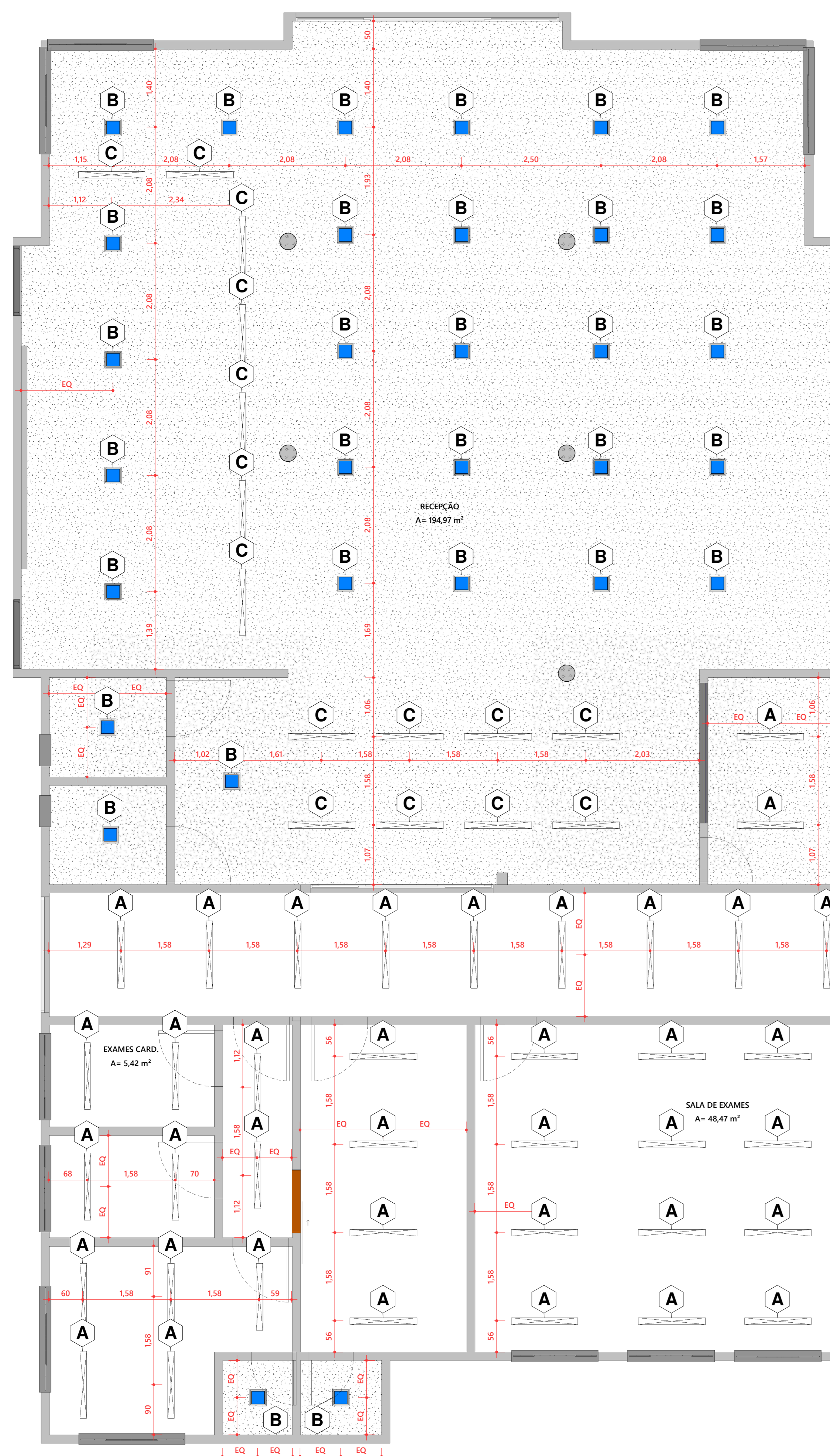
LUMINOTÉCNICO TÉRREO ESCALA: 1:50
