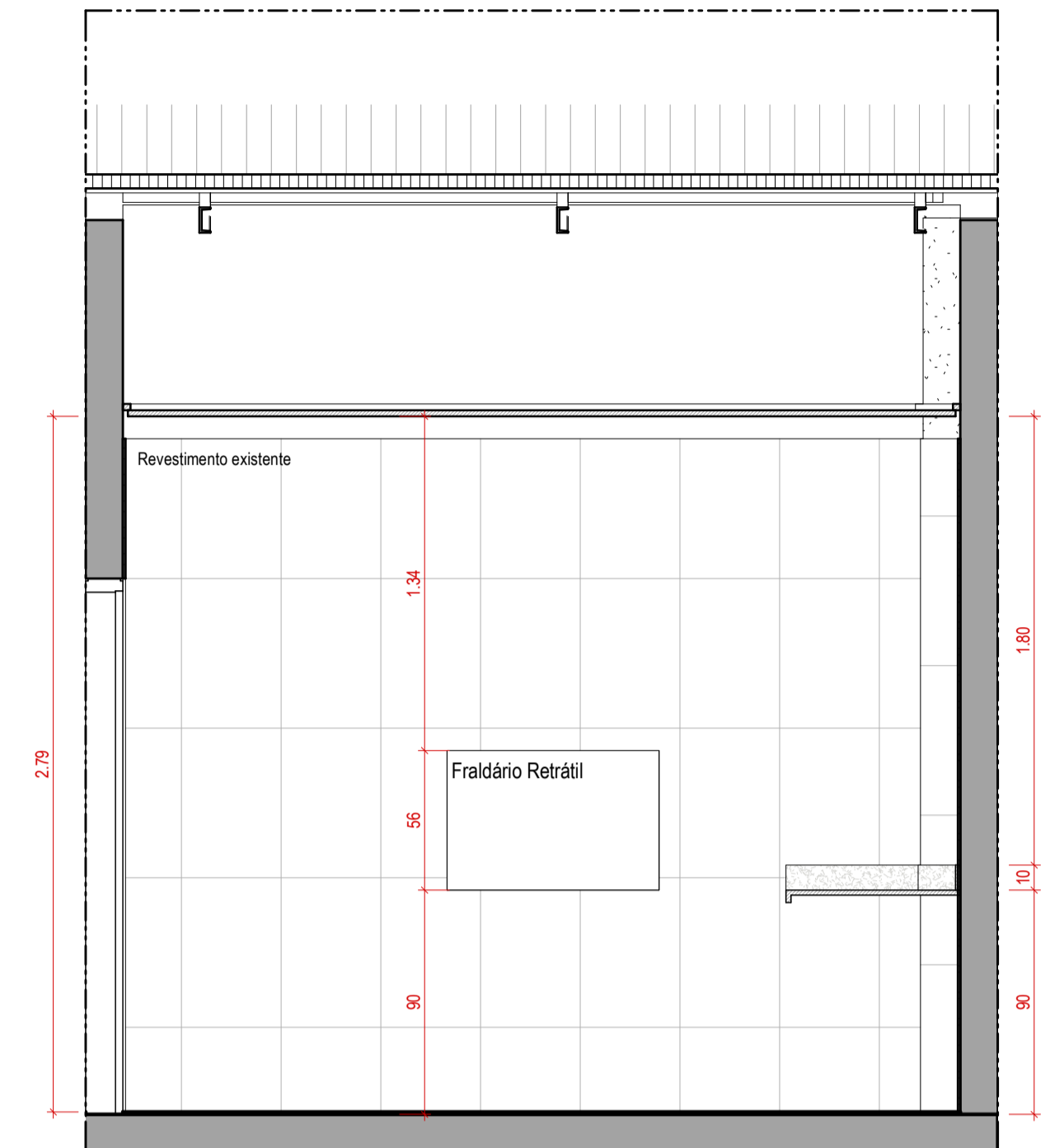
VISTA B - Fraldário ESCALA 1:25
