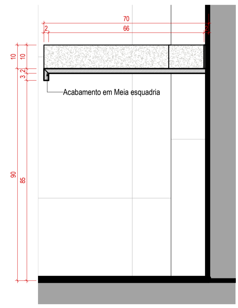
6 | Det. Bancada Fraldário. ESCALA 1:10
