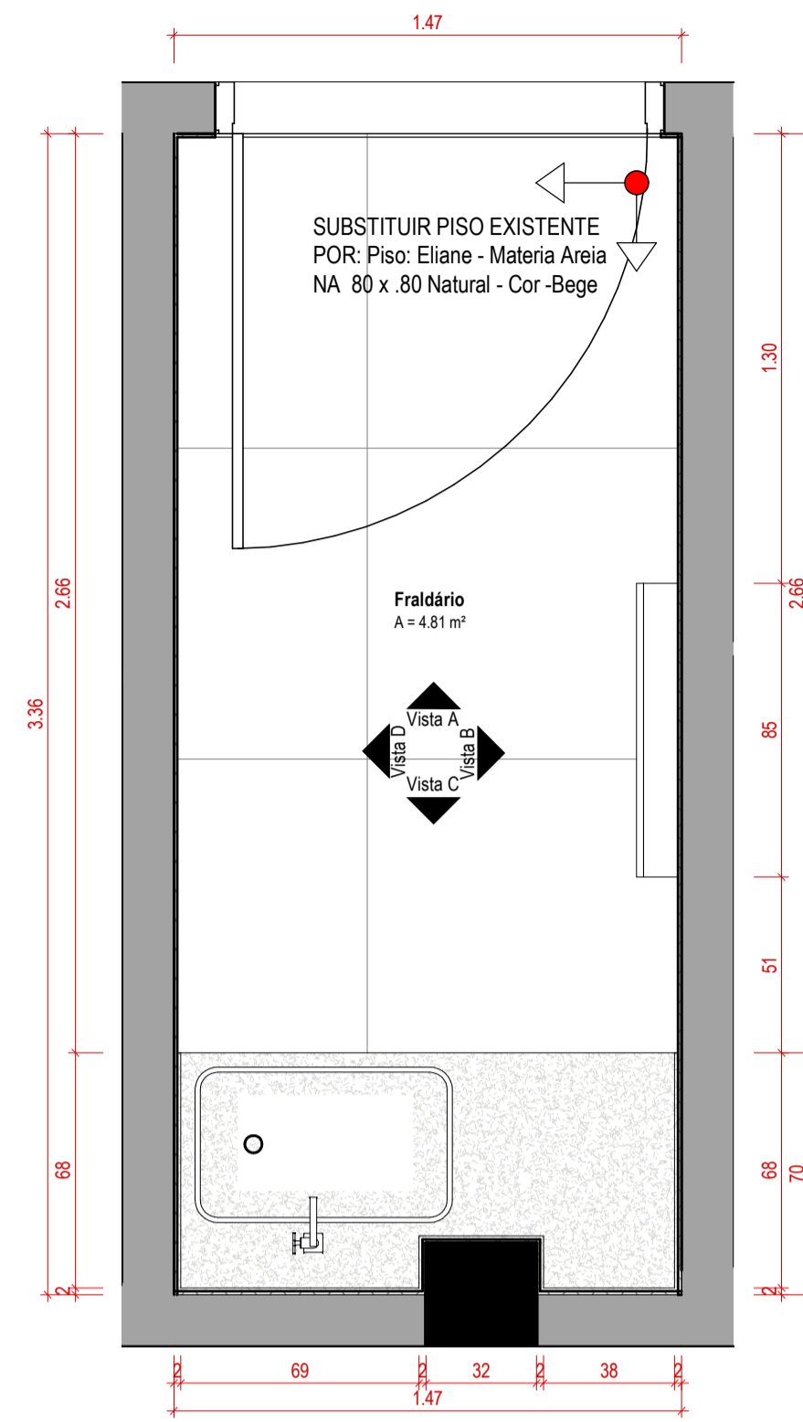
Planta Fraldário ESCALA 1:20
