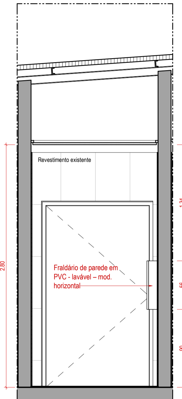
VISTA A - Fraldário ESCALA 1:25
