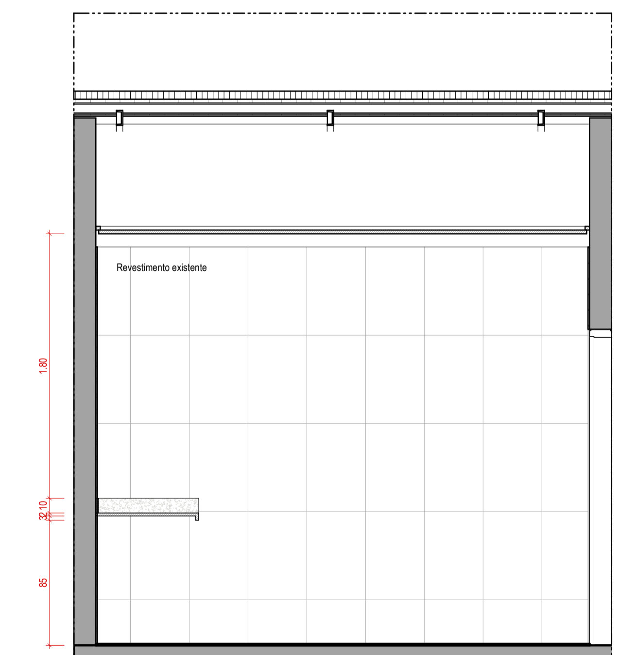
5 | VISTA D - Fraldário ESCALA 1:25
