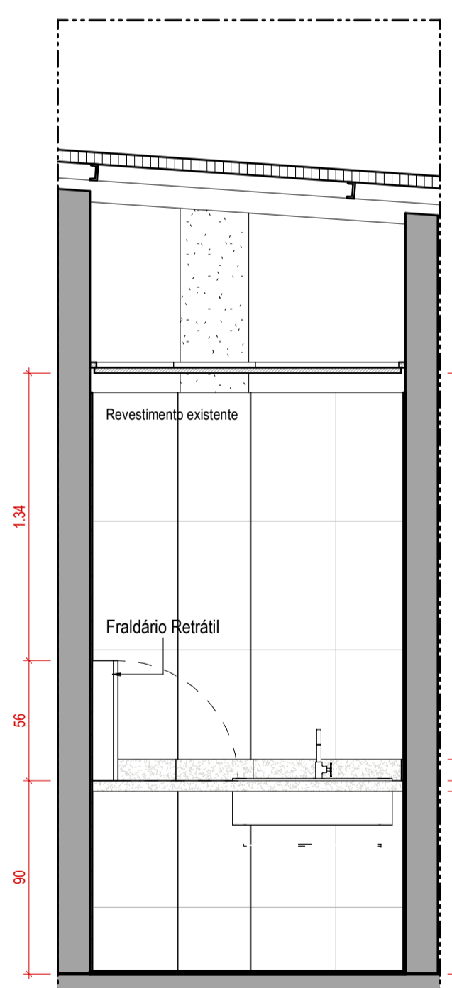
2 | VISTA C - Fraldário ESCALA 1:25
