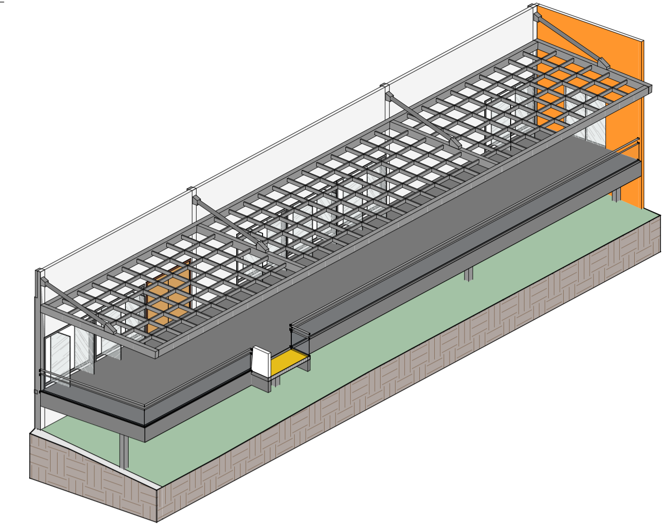
5 Estrutura Pergolado
