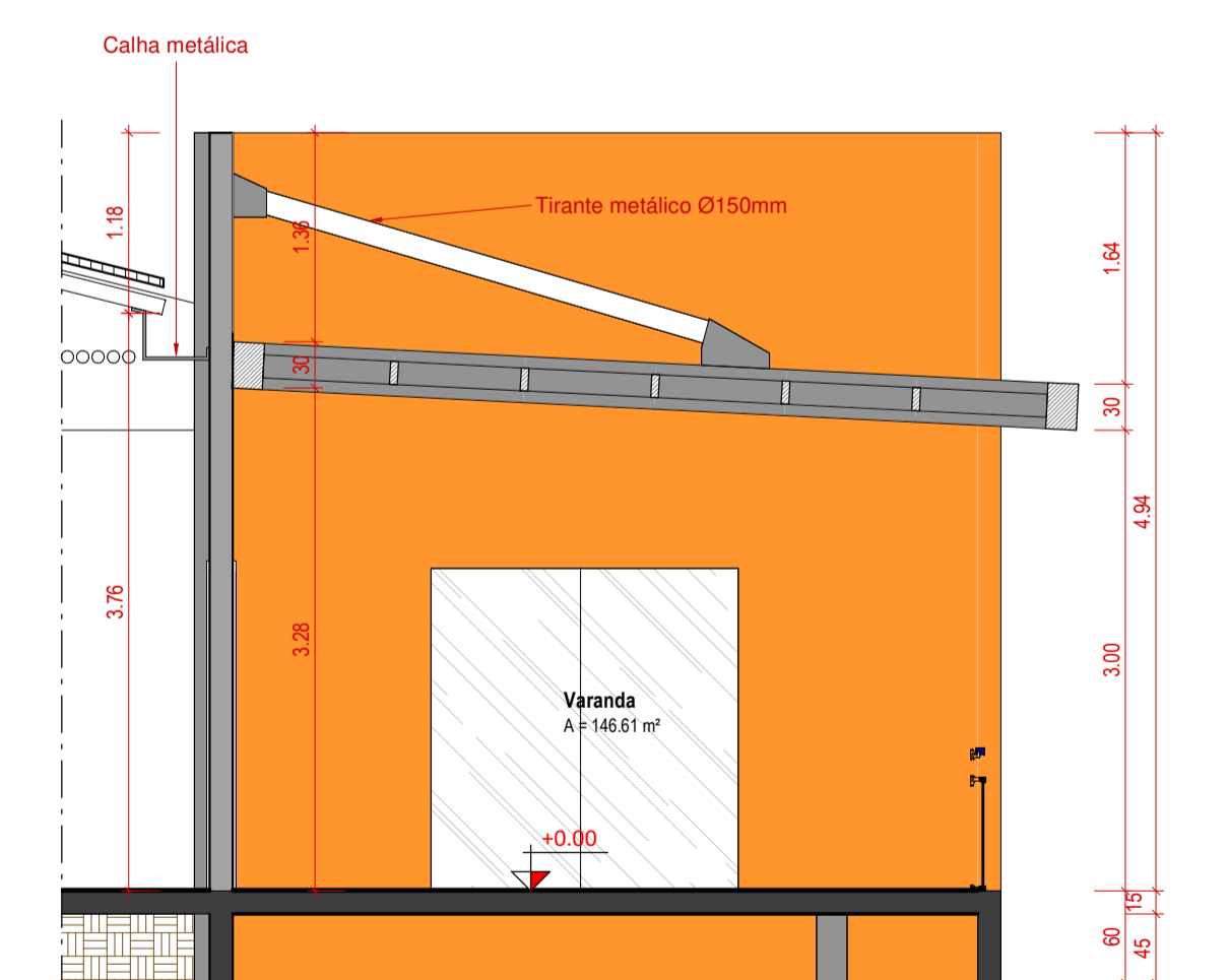
J CORTE J - Pergolado 1 : 50
