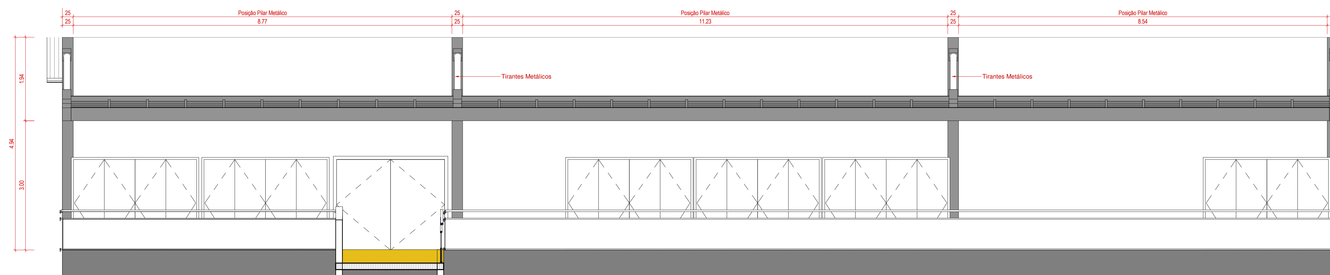
3 VISTA PERGOLADO - FACHADA NORDESTE 1 : 50
